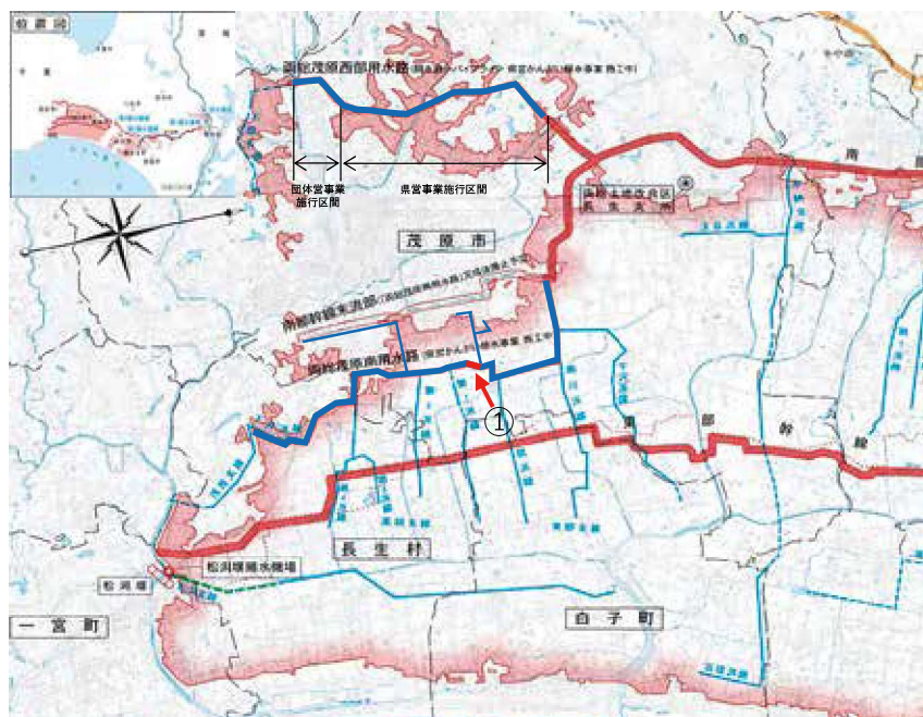
「両総茂原南地区」支線用水路工事 (6の13) 施工予定路線
